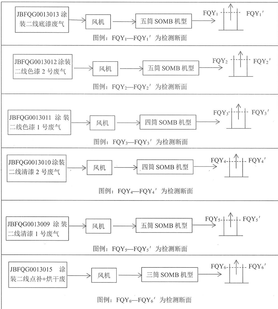
图3 有组织废气采样点示意图
