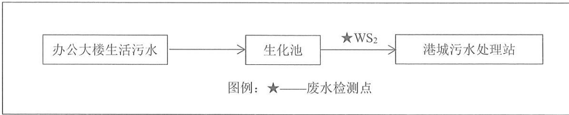
图2 废水采样点示意图(续)
