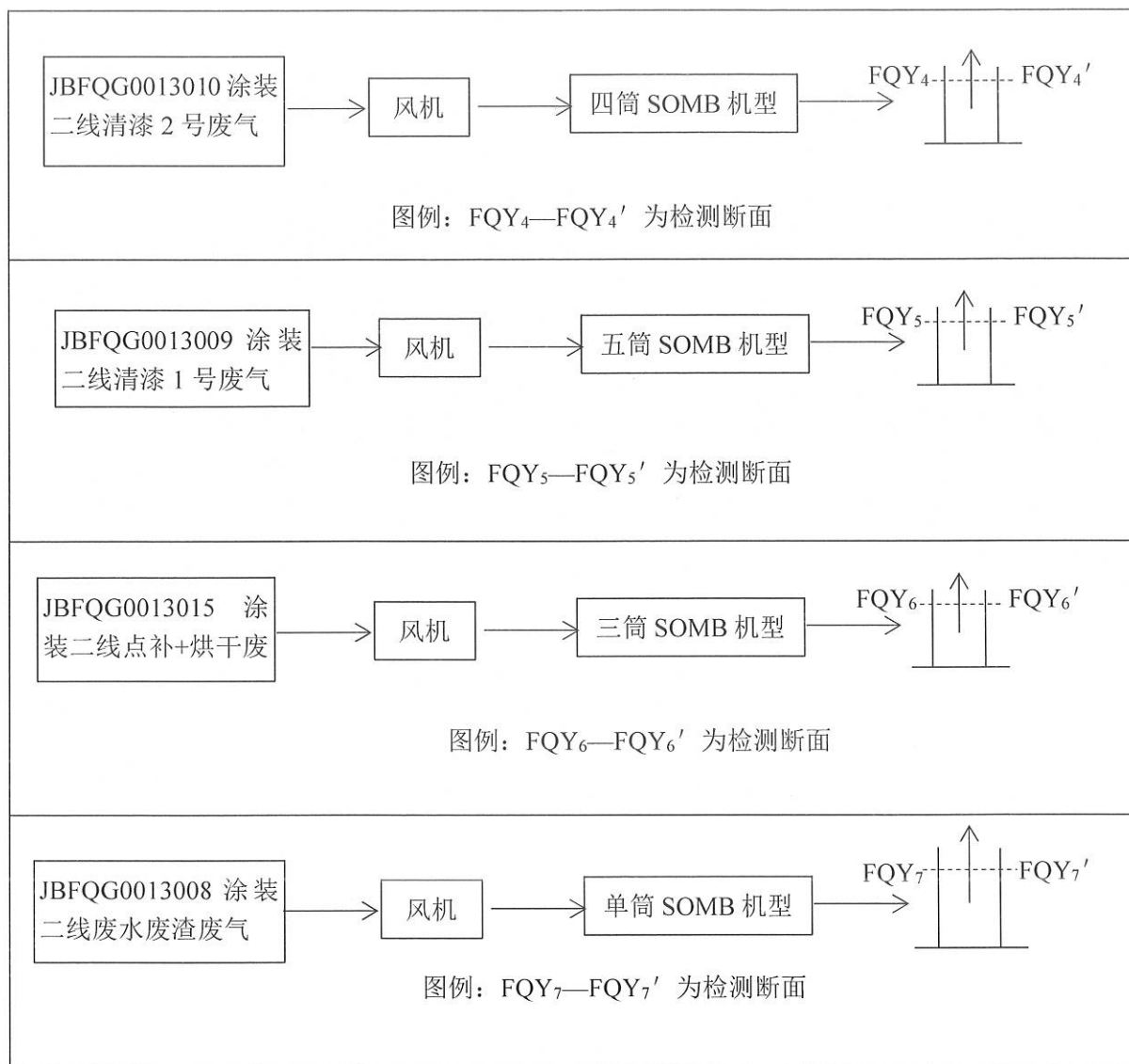
图3 有组织废气采样点示意图(续)
