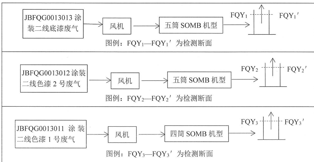
图3 有组织废气采样点示意图
